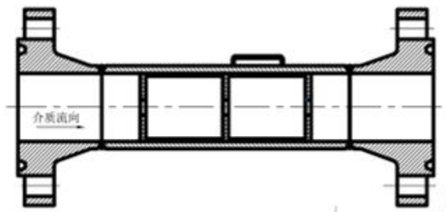
多级带法兰限流孔板
