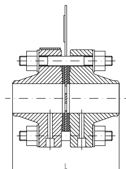
单级法兰限流孔板
