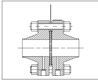
基本式结构 F
