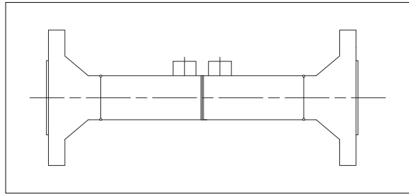
管道式（管嘴取压）G
