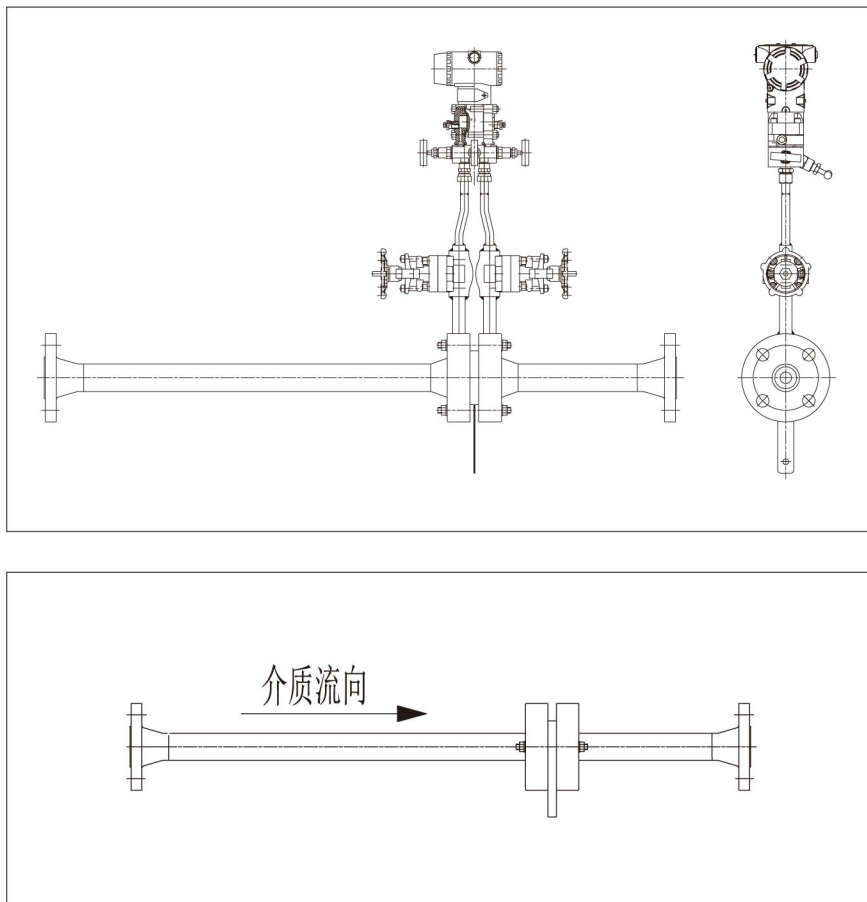
外形图
