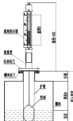
UHC 顶装磁性浮子式液位计 (普通型)
