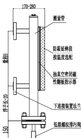
UHC 侧装磁性浮子式液位计
