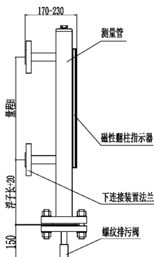
UHC 侧装磁性浮子式液位计
